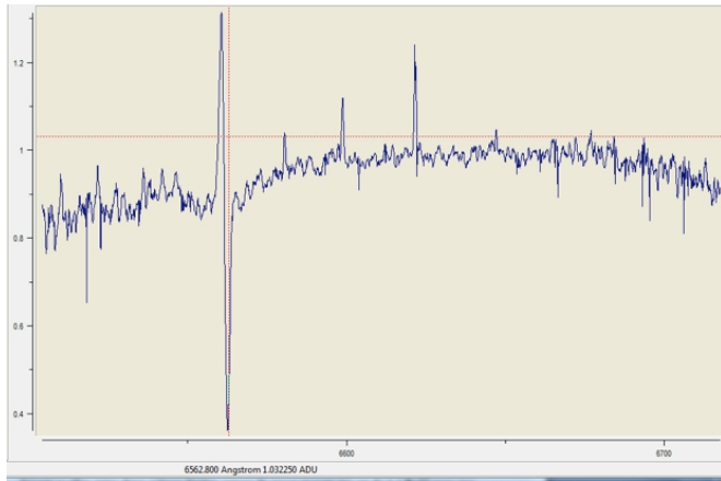
FIGURE 7 – Emission de la raie H_\alpha au maximum de la phase Blazhko. Le trait rouge indique la longueur de H_\alpha au laboratoire
