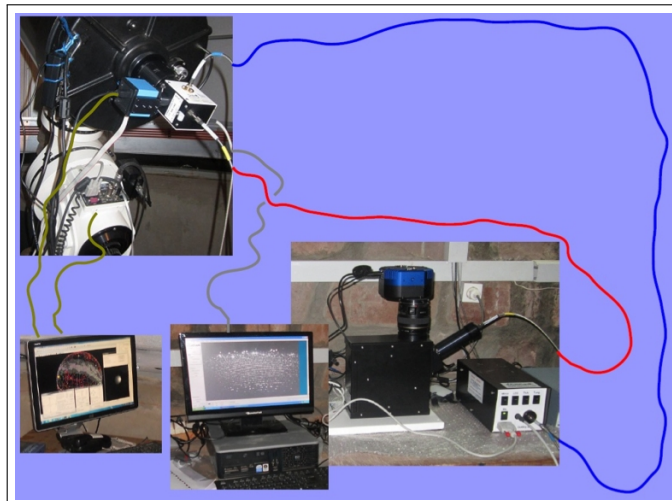
FIGURE 6 – Montage du Spectrographe eShel
