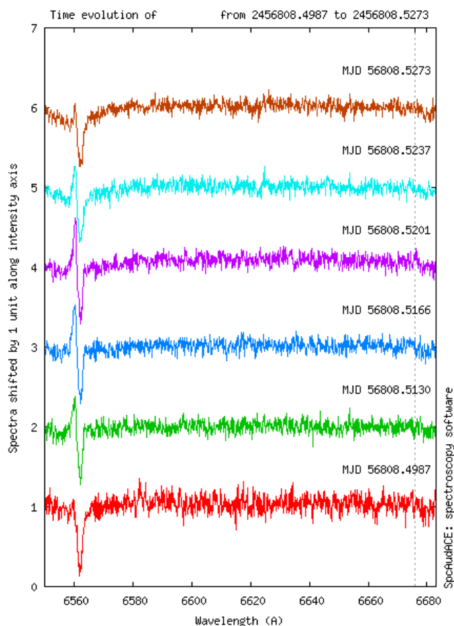
FIGURE 1 – Série spectrale autour du maximum avec la raie He I 6678 Å en émission (spectre violet).
