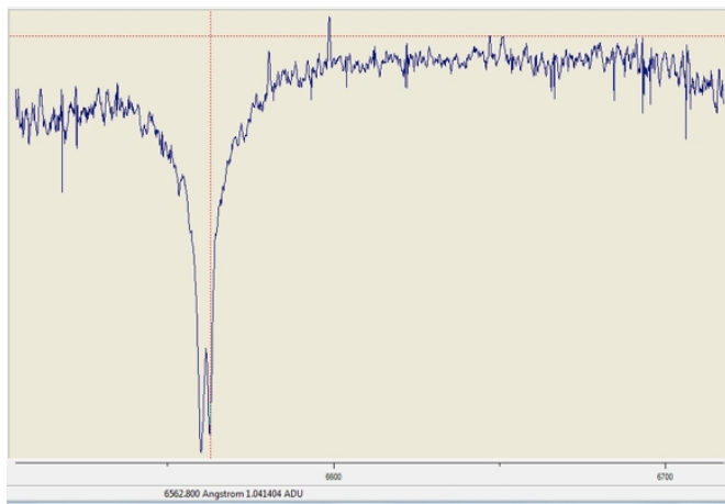
FIGURE 8 – Dédoublement de la raie H_\alpha . Le trait en rouge indique la longueur d'onde de H_\alpha au laboratoire
