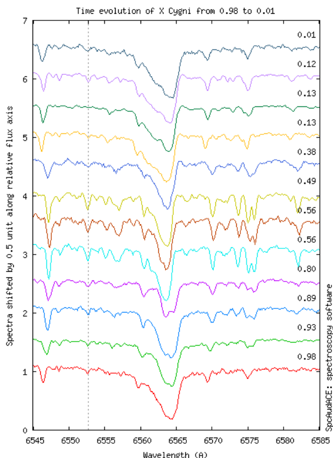
FIGURE 3 – Série de spectres de X Cygni réalisée durant le 3ème trimestre 2013 par B. MAUCLAIRE. Un repère sur une raie tellurique montre que la calibration est stable.
