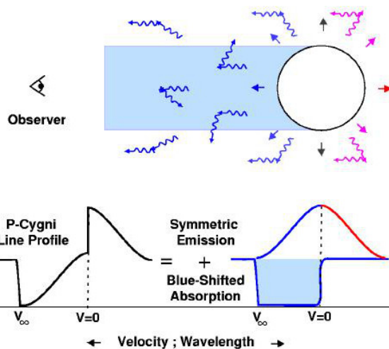
FIGURE 4 – Formation d'une raie de type P-Cygni [OWOCKI 2014].
