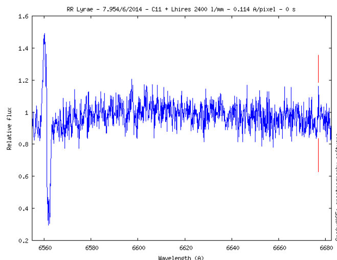
FIGURE 2 – Spectre du 7 juin 2014 montrant l'émission de la raie He I 6678 Å.
